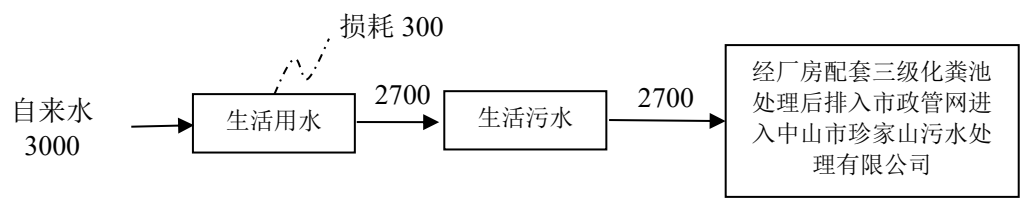
图 1 全厂水平衡图 (单位: t/a)
