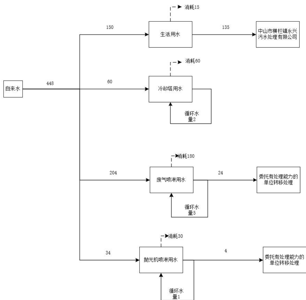
图 2-1 项目水平衡情况图 (m³/a)
