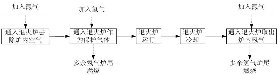
图 9 退火炉工艺流程图
