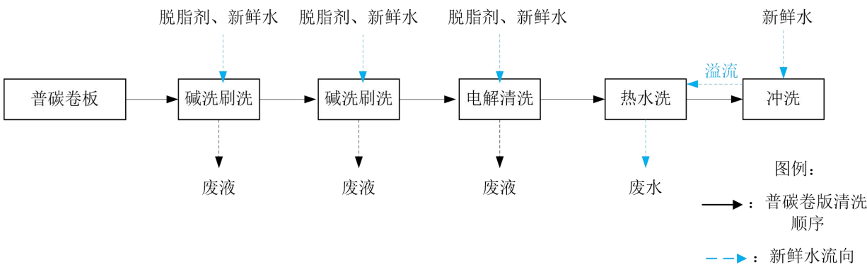
图 8 碱洗脱脂、清洗工艺流程图
