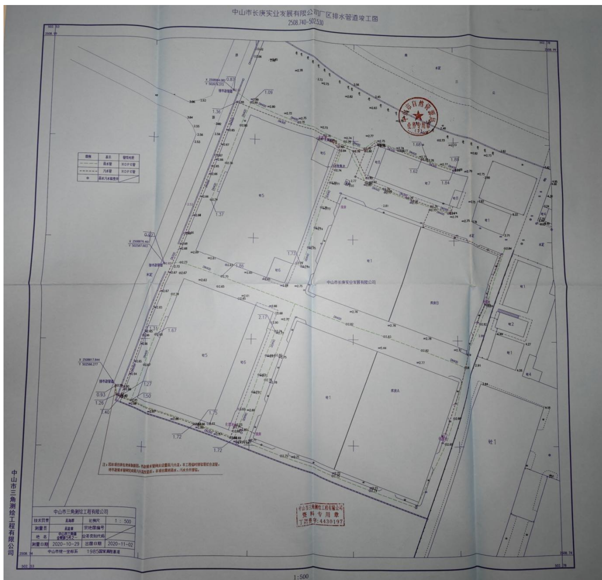
图 6.7-1 应急池、雨水管网及阀门情况分布图
