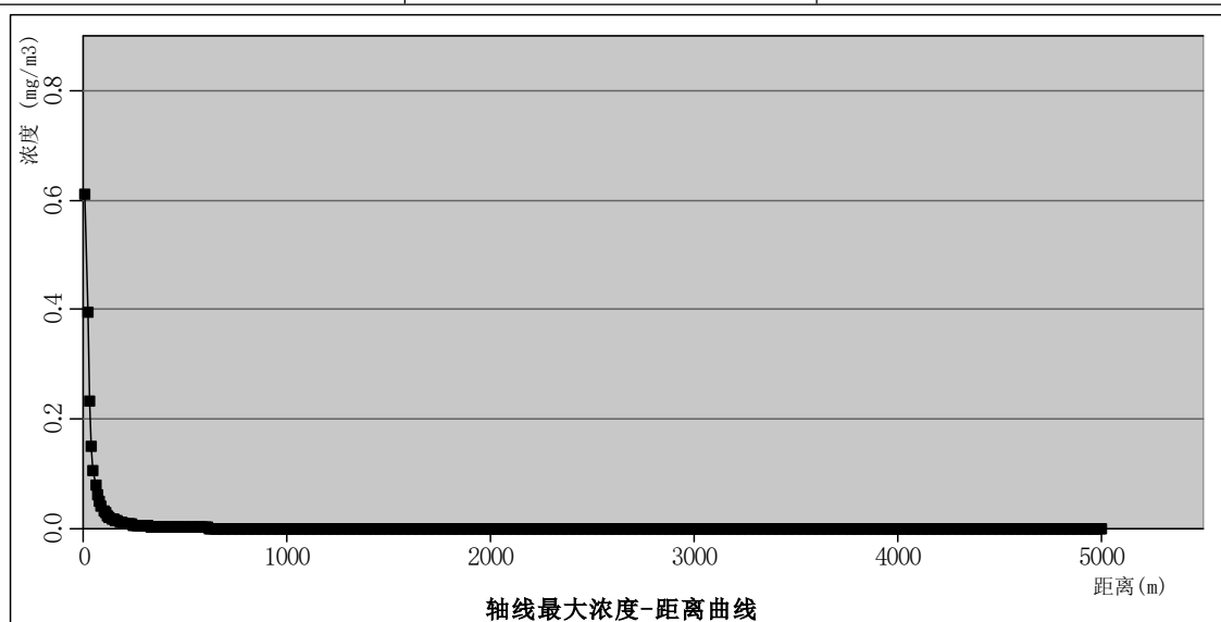
图 6.6-3 硫酸泄漏轴线/质心最大浓度图（最常见气象条件下）
