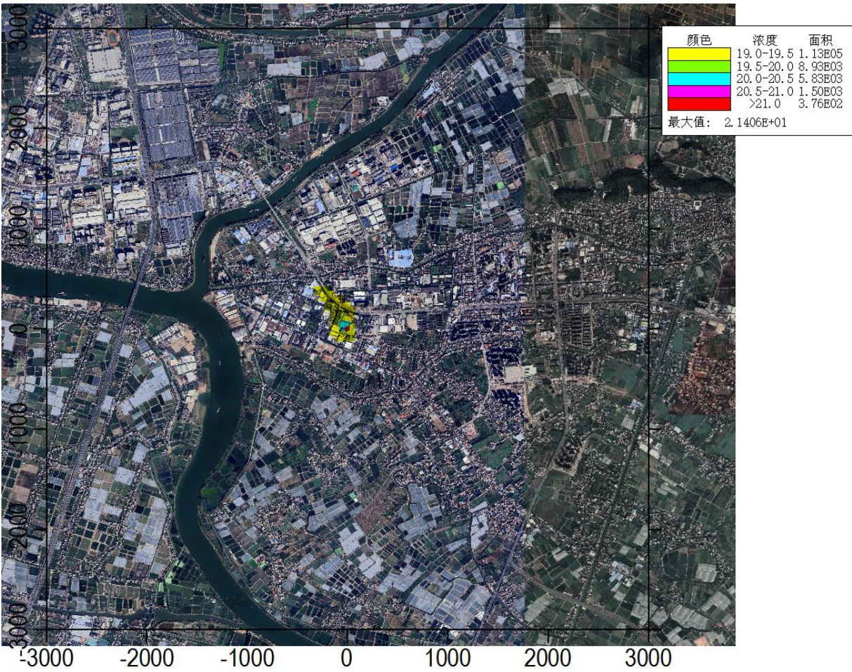
图 6.1-15 正常排放 \text{PM}_{2.5} 年平均浓度预测值分布图
