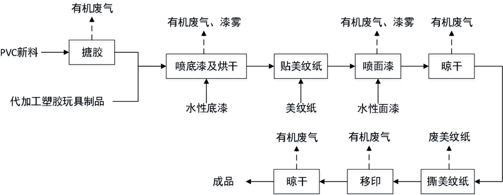
图 2 工艺流程图
