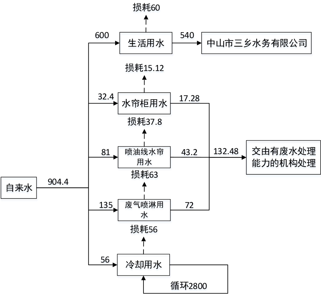
图 1 项目水平衡图（单位： t/a）
