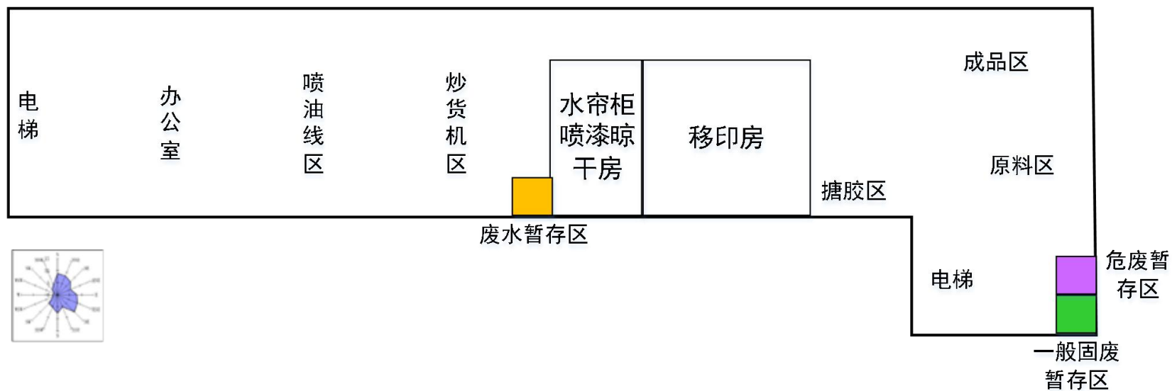
附图 9-1 车间平面布置图（三层）
