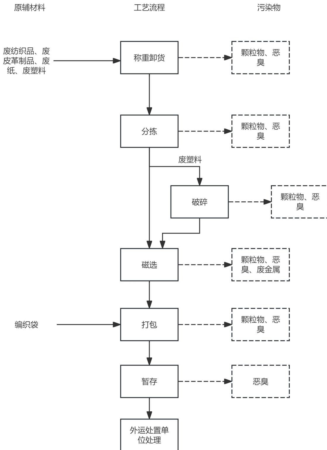
图 2-2 工艺流程及产污环节图
