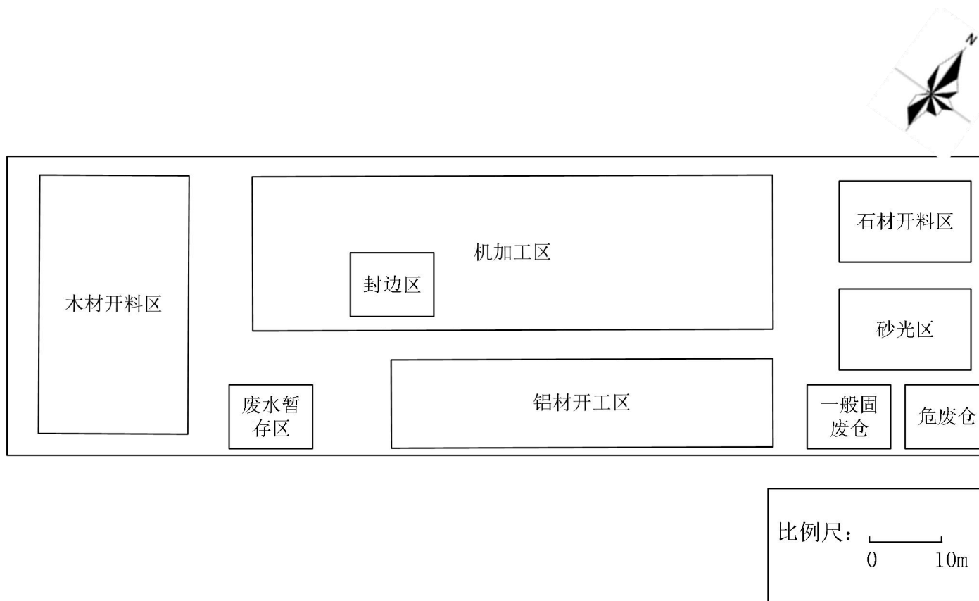
附图 3-1、项目一楼布置图
