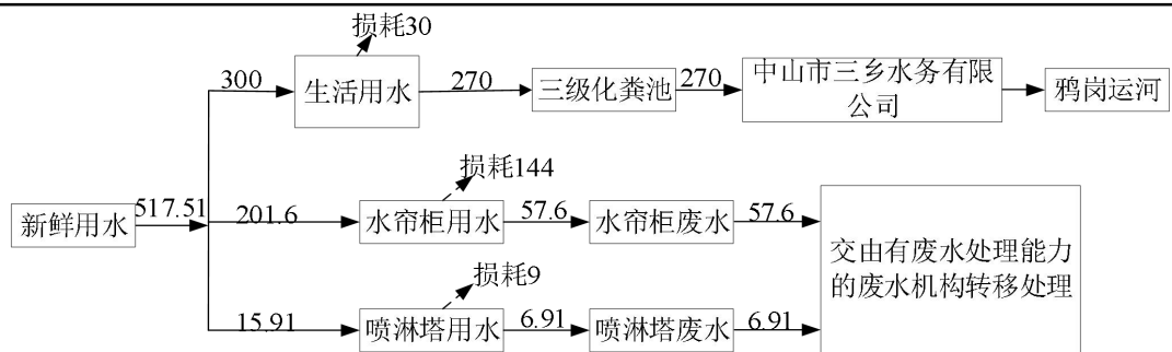
图 1-1 项目水平衡图(t/a)
