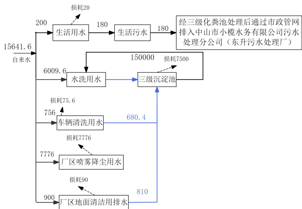
图 1：全厂水平衡图（单位：t/a）
