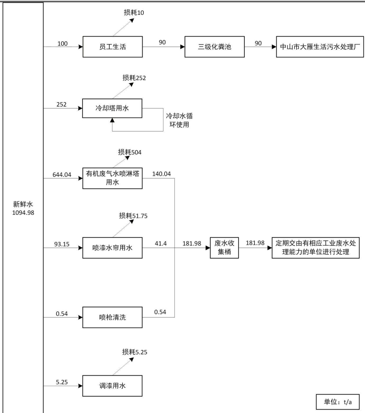
图 1 项目水平衡图
