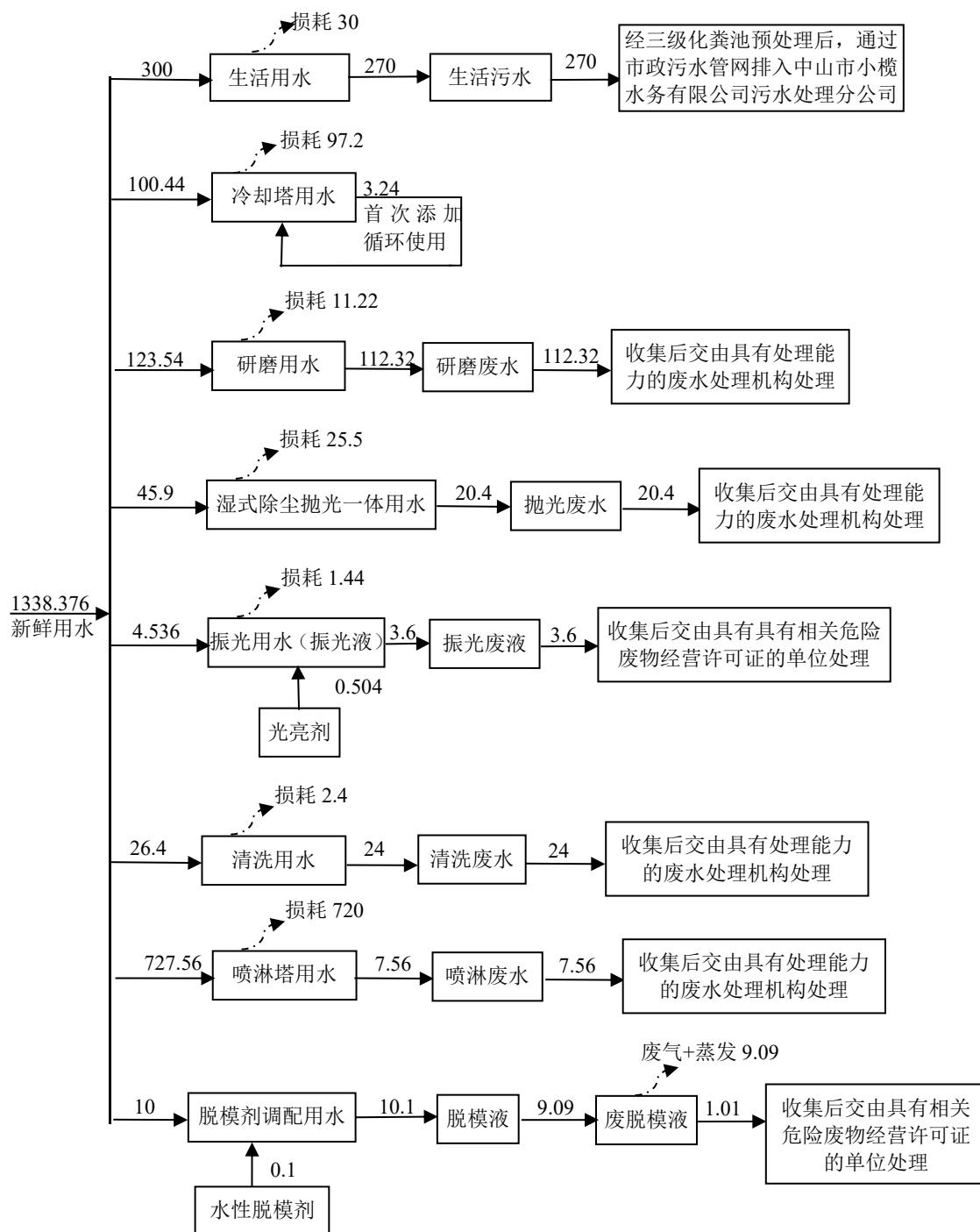
图 2-1 项目水平衡图 (t/a)
