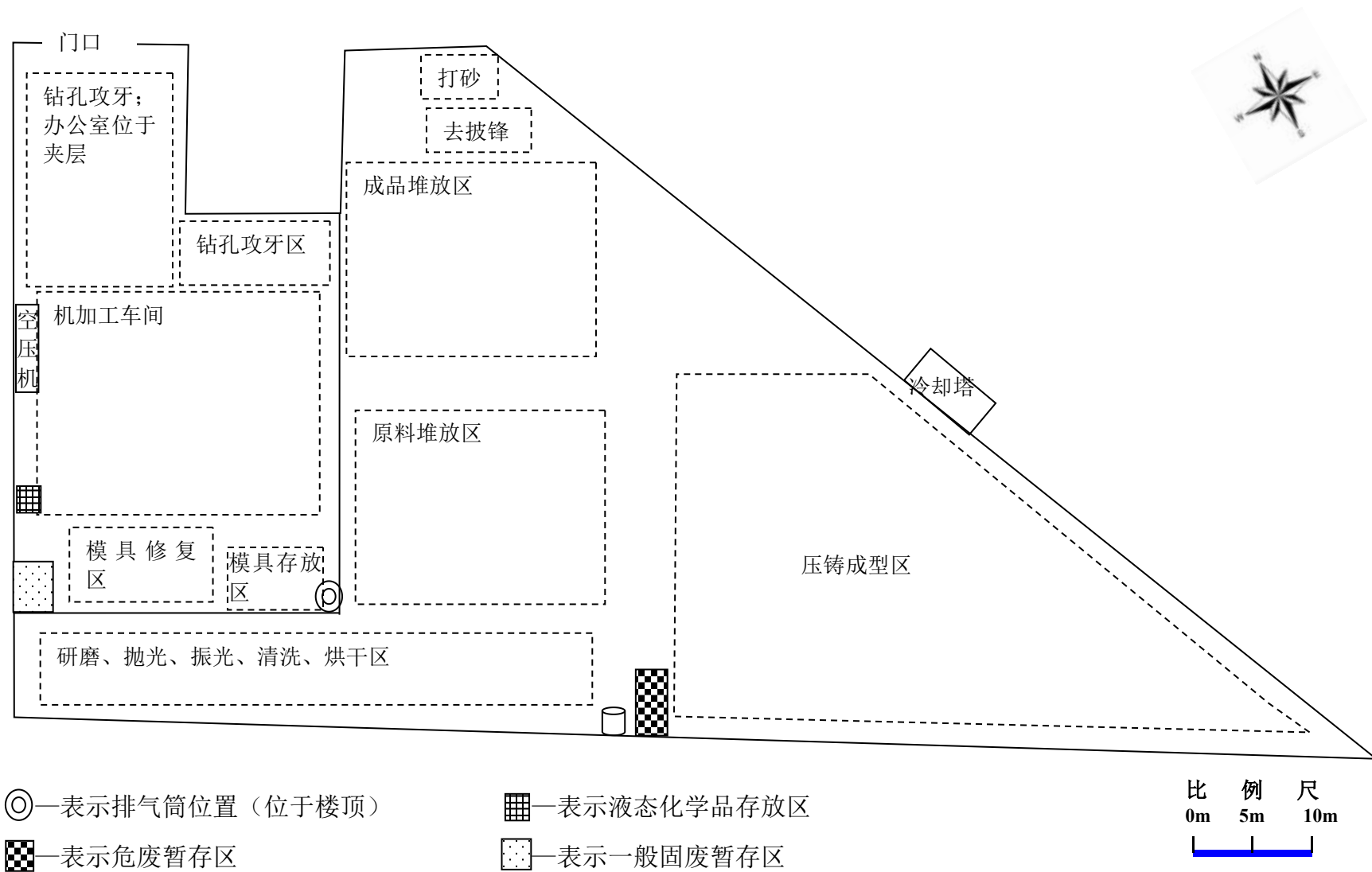
附图 2 项目平面布置示意图
