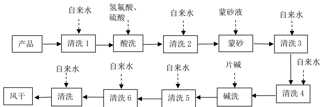
附图 2-1 本项目自动蒙砂清洗流程图
