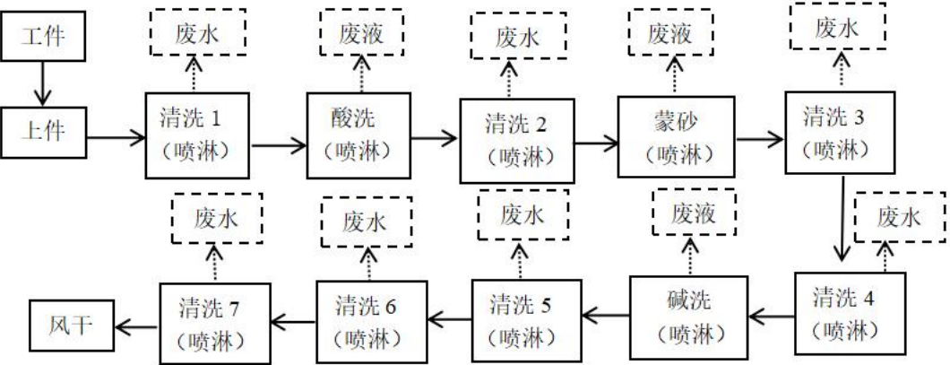
图 2-6 自动蒙砂生产线装置连接图
