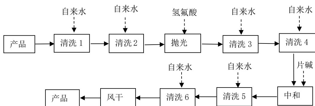
附图 2-2 本项目自动抛光清洗流程图
