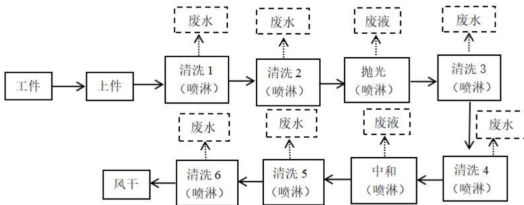
图 2-7 抛光生产线装置连接图
