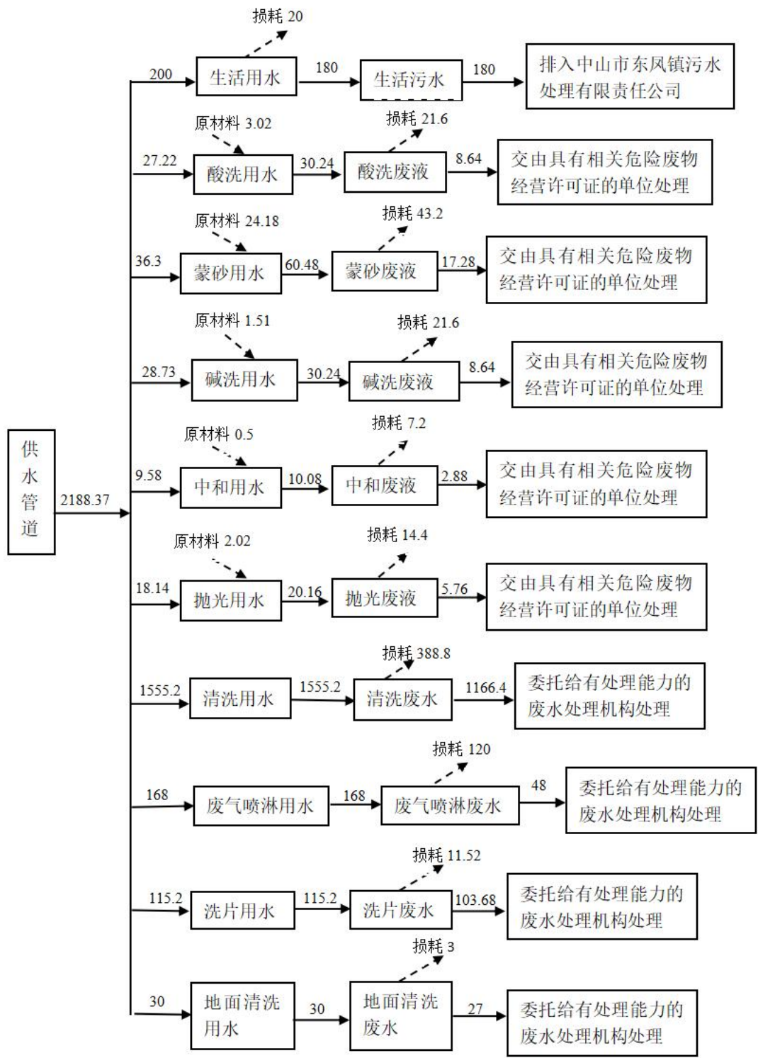
项目水平衡图：
