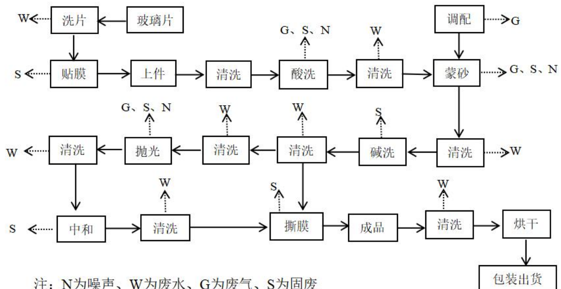
图 2-5 本项目蒙砂玻璃生产工艺流程及产污环节图
